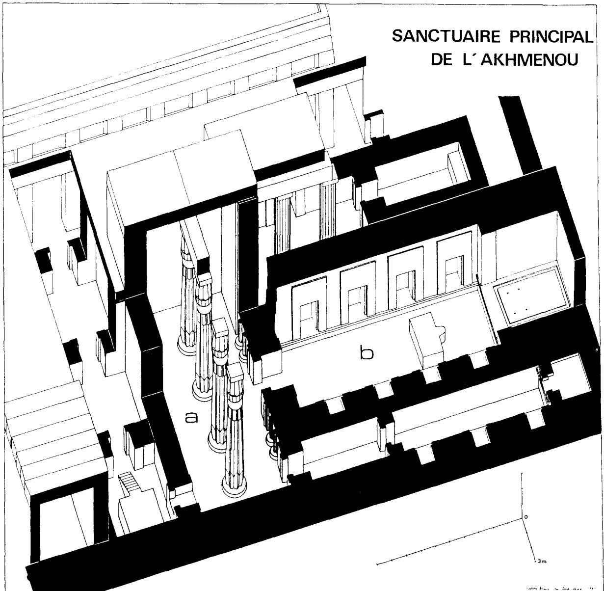
Axonométrie des salles du «Jardin botanique». État initial. (Dessin : Nathalie Beaux et Jean-Claude Golvin.) a. Vestibule. b. Sanctuaire.
